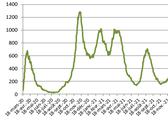
Hospitalisation conventionnelle
